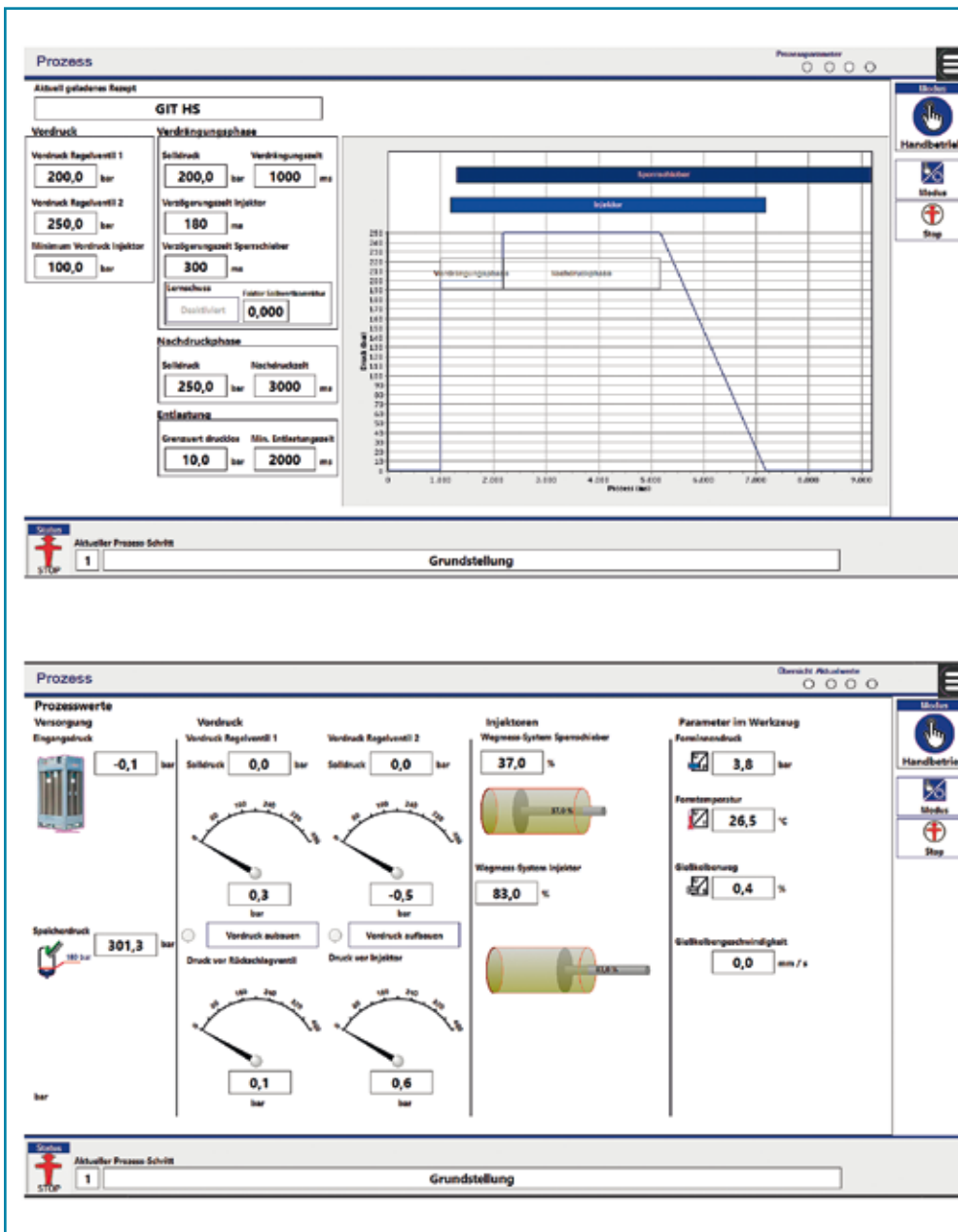
Bild 6: Bedienoberfläche des Tablet-PCs zur Steuerung des neuen Gasinjektionssystems: Eingabe der für die Gasinjektion relevanten Prozessparameter (oben), Echtzeitüberwachung des Systems mit verschiedenen Gasdruckniveaus, der Position des Gasinjektors und des Sperrschiebers sowie Sensorsignalen (unten).
