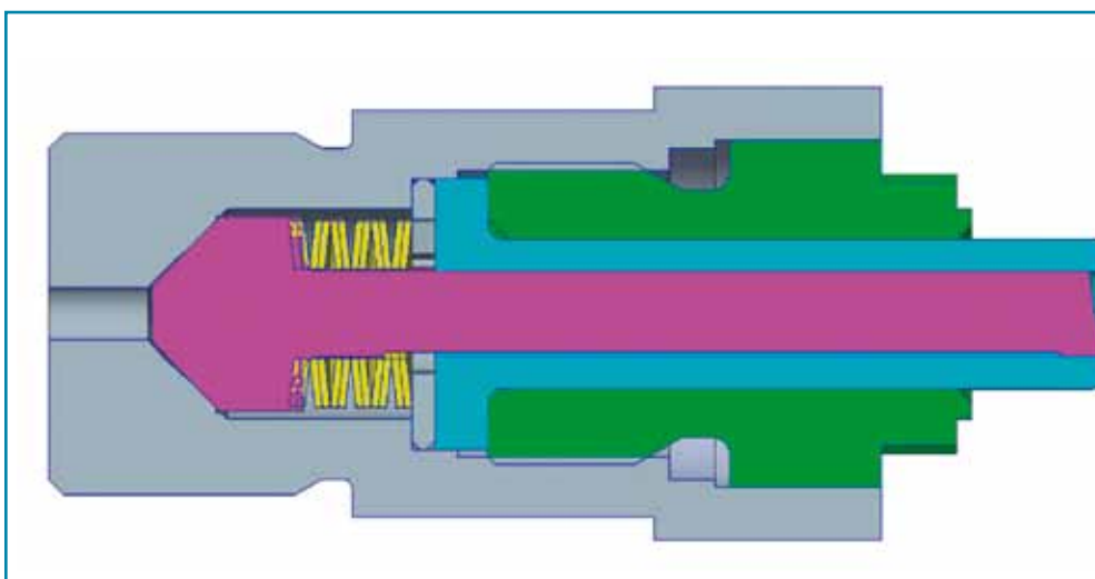
Figure 7: Neu entwickelter Gasinjektor mit Sonderwerkstoffen im Bereich der mit flüssigem Metall in Kontakt tretenden Bereiche Hülse (blau) und Nadel (magenta)
